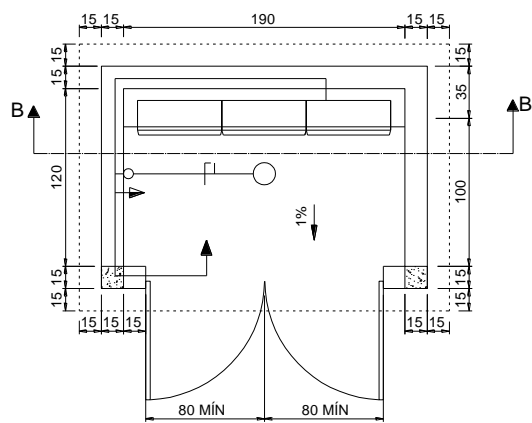
PLANTA BAIXA
